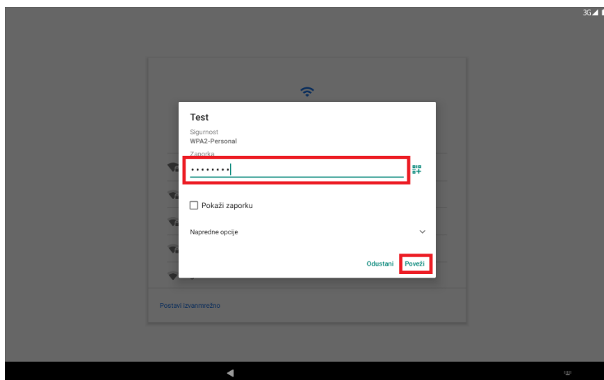
Slika 6. Upisivanje lozinke
